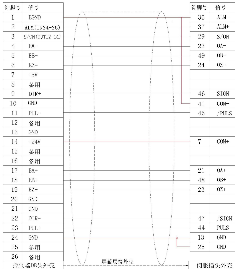
ZMC306N 控制器和松下 A5 伺服驱动器高速差分脉冲口接线参考
