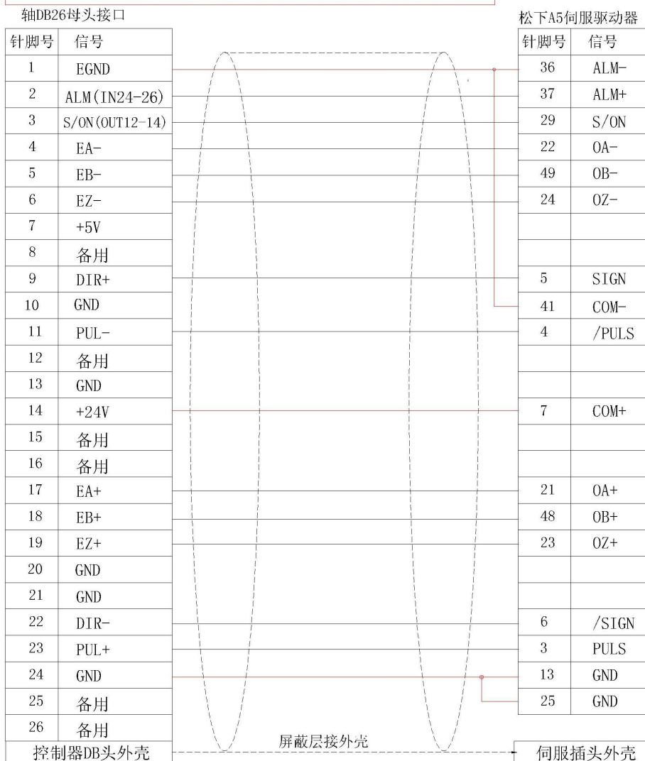
ZMC306N 控制器和松下 A5 伺服驱动器低速差分脉冲口接线参考
