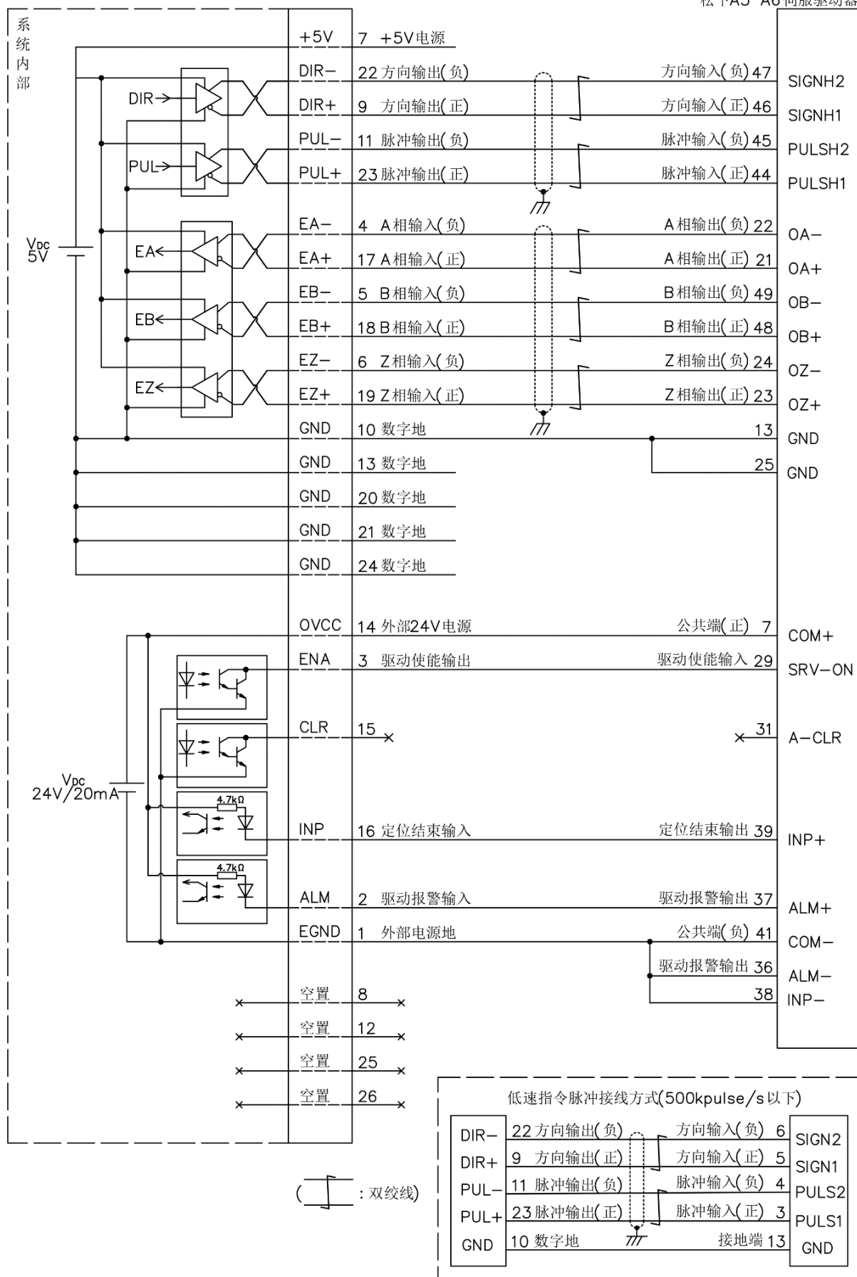
松下A5 A6伺服驱动器
