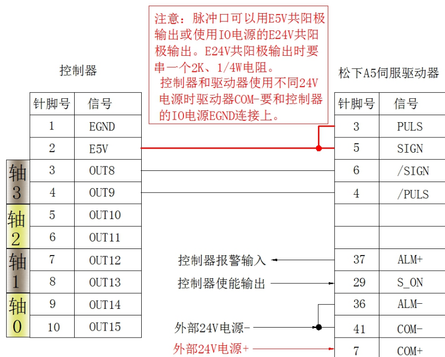
与松下 A5 单端接线参考
