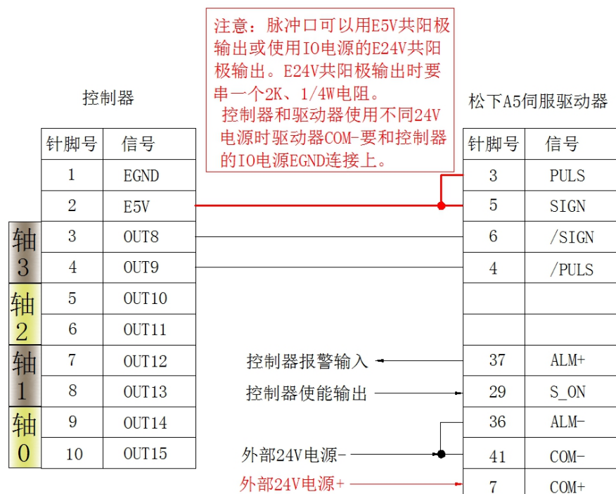
与松下 A5 单端接线参考
