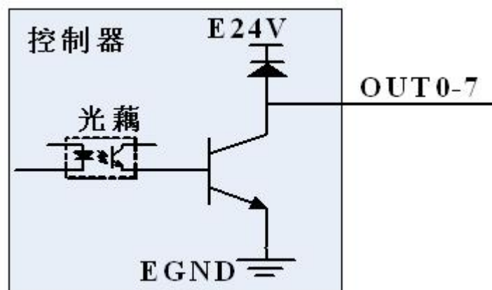
输出电路
