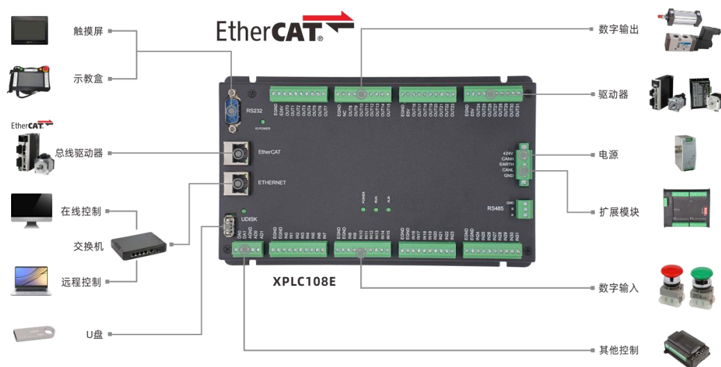
典型连接配置图
